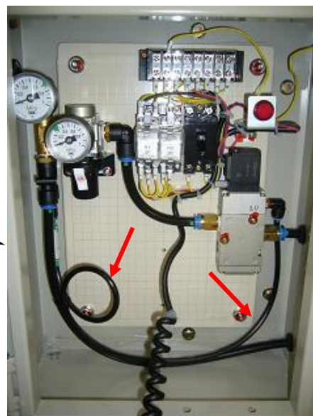
(コントロールボックス内部配管) 赤矢視は誤配管部分を示す
